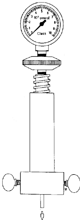
2. mynd: Þrýstímælir fyrir kork- eða plasttappa
