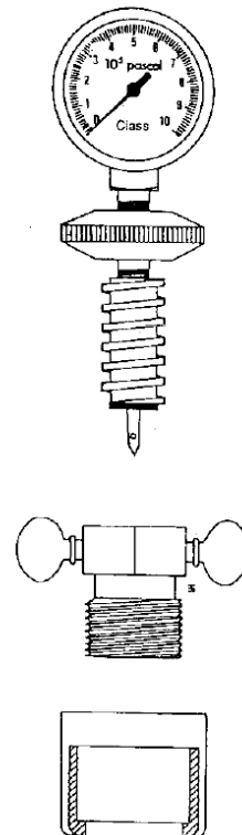
1. mynd — Þrýstímælir fyrir málm-tappa
