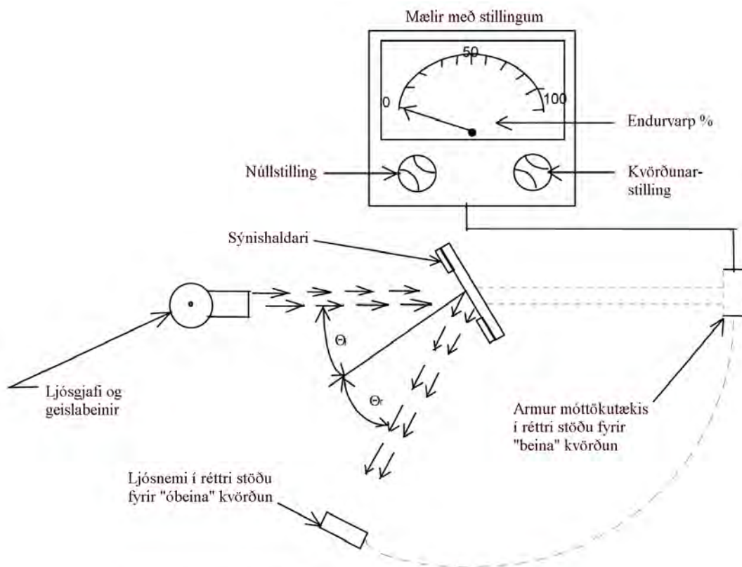
Mynd 4: Almenn teikning af endurvarpsmæli sem sýnir báðar kvörðunaraðferðir
