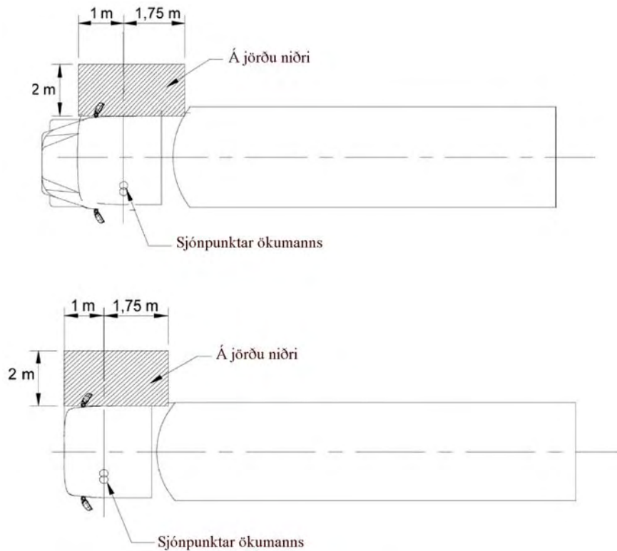
Myndir 10a og 10b Sjónsvið nálægðarspegils í flokki V
