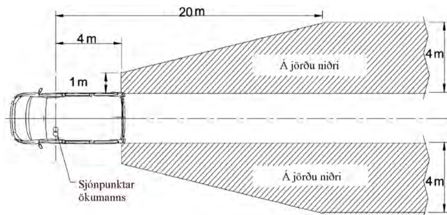
Mynd 8 Sjónsvið spegla í flokki III
