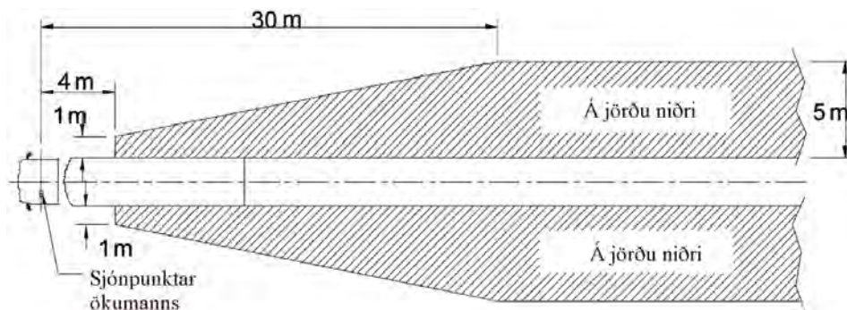
Mynd 7: Sjónsvið spegla í flokki II
