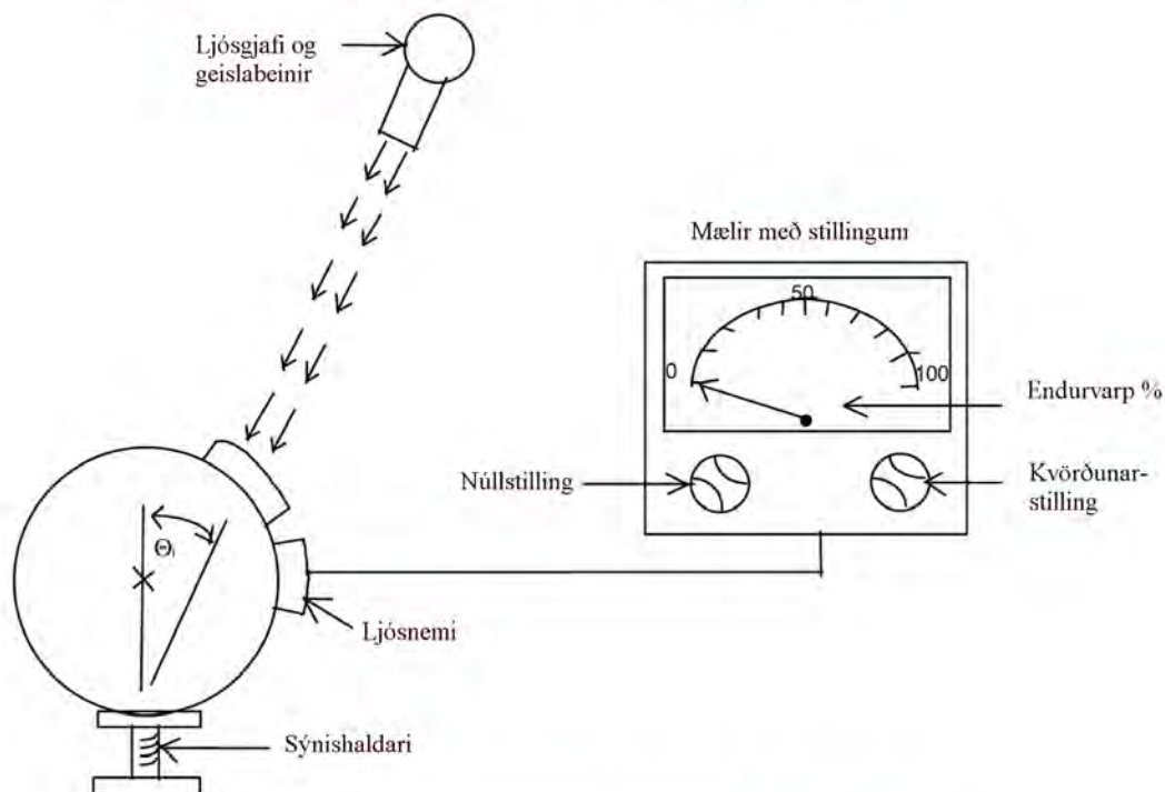
Mynd 5: Almenn teikning af endurvarpsmæli með ljósmælikúlu í móttökutæki
