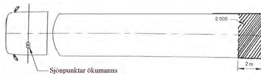
Mynd 12 Sjónsvið búnaðar til að auka sjónsvið á afturhluta ökutækisins
