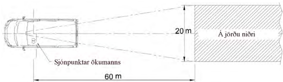
Mynd 6: Sjónsvið spegils í flokki I
