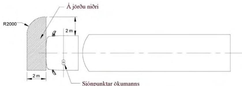
Mynd 11 Sjónsvið framsýnispegils í flokki VI
