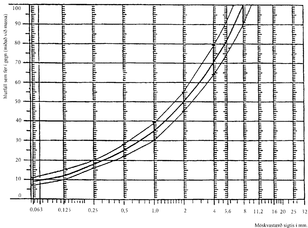
Sáldurferill steinefna í malbiksblöndunni með vikmörkum
